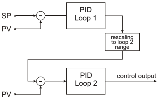
Fig. 21. Cascade control
