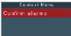
Fig. 13. Context menu
